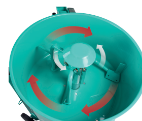
Sistema di inversione del senso di rotazione delle pale. Permette di disintegrare eventuali grumi e di riprendere la mescolazione normale senza interventi manuali diretti.
